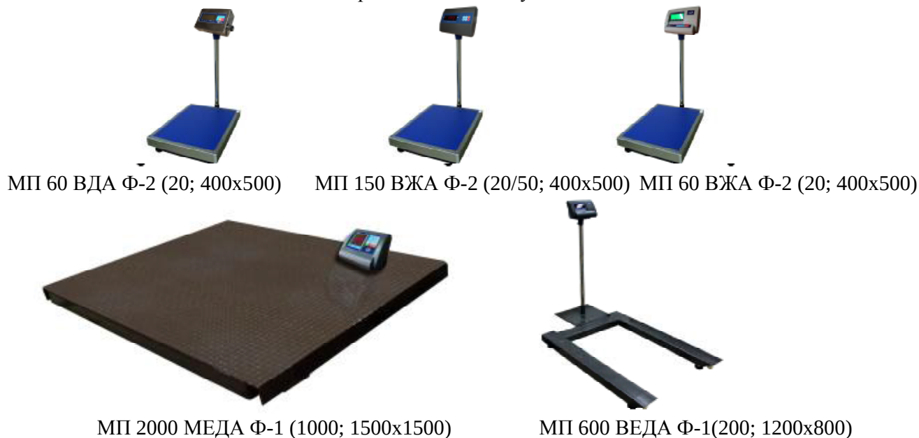
Рисунок 1 — Общий вид весов
